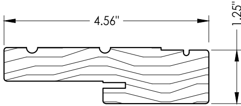
20 HEAD & SIDE Jamb
