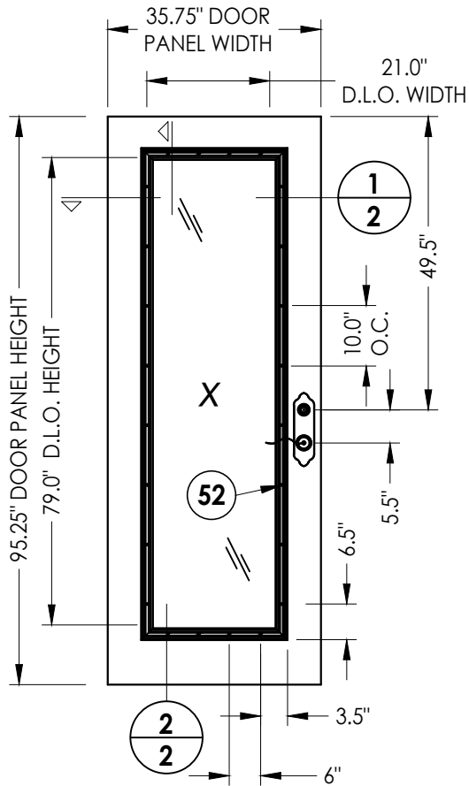
40 DOOR PANEL
