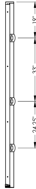
STRIKE JAMB
